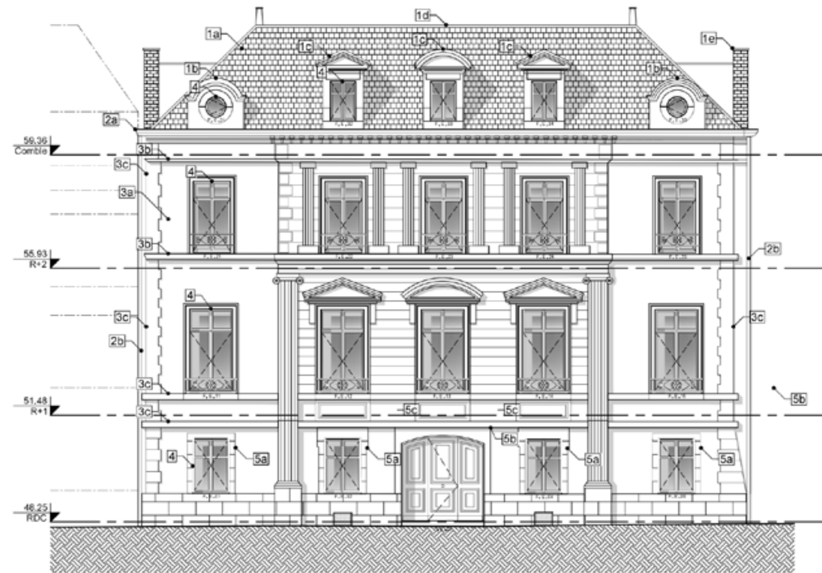
FAÇADE EST
